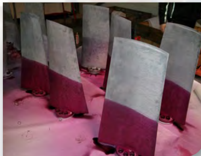
Prüfung Laufradschaufeln mittels Farbeindringverfahren
