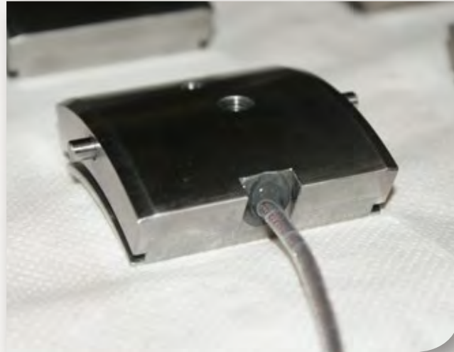
Gleitlagersegment mit PT100 (Temperaturüberwachung)
